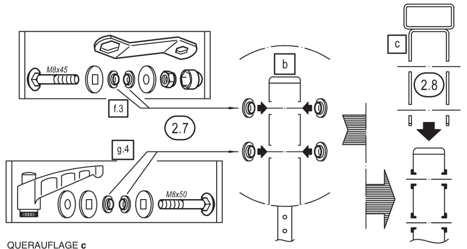
QUERAUFLAGE c
