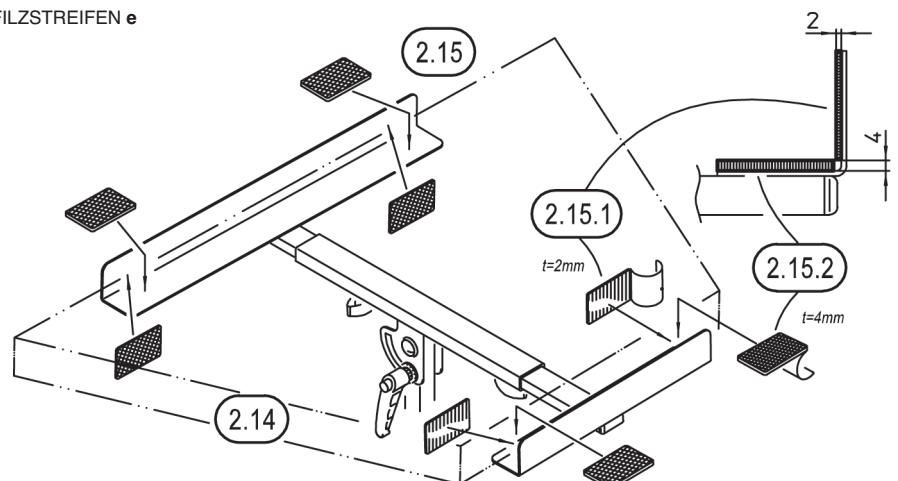
FILZSTREIFEN e
