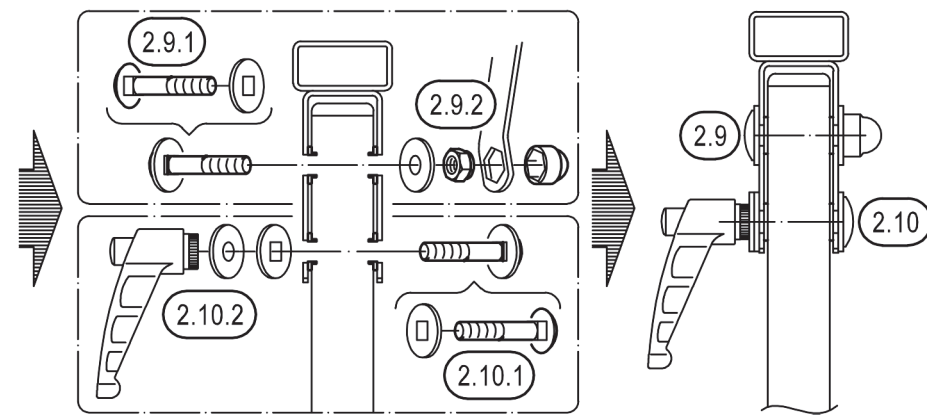
VERSTELLBÜGEL d
